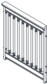
E Crib End (Left) / Lit Fin (Gauche) ( x1 )
