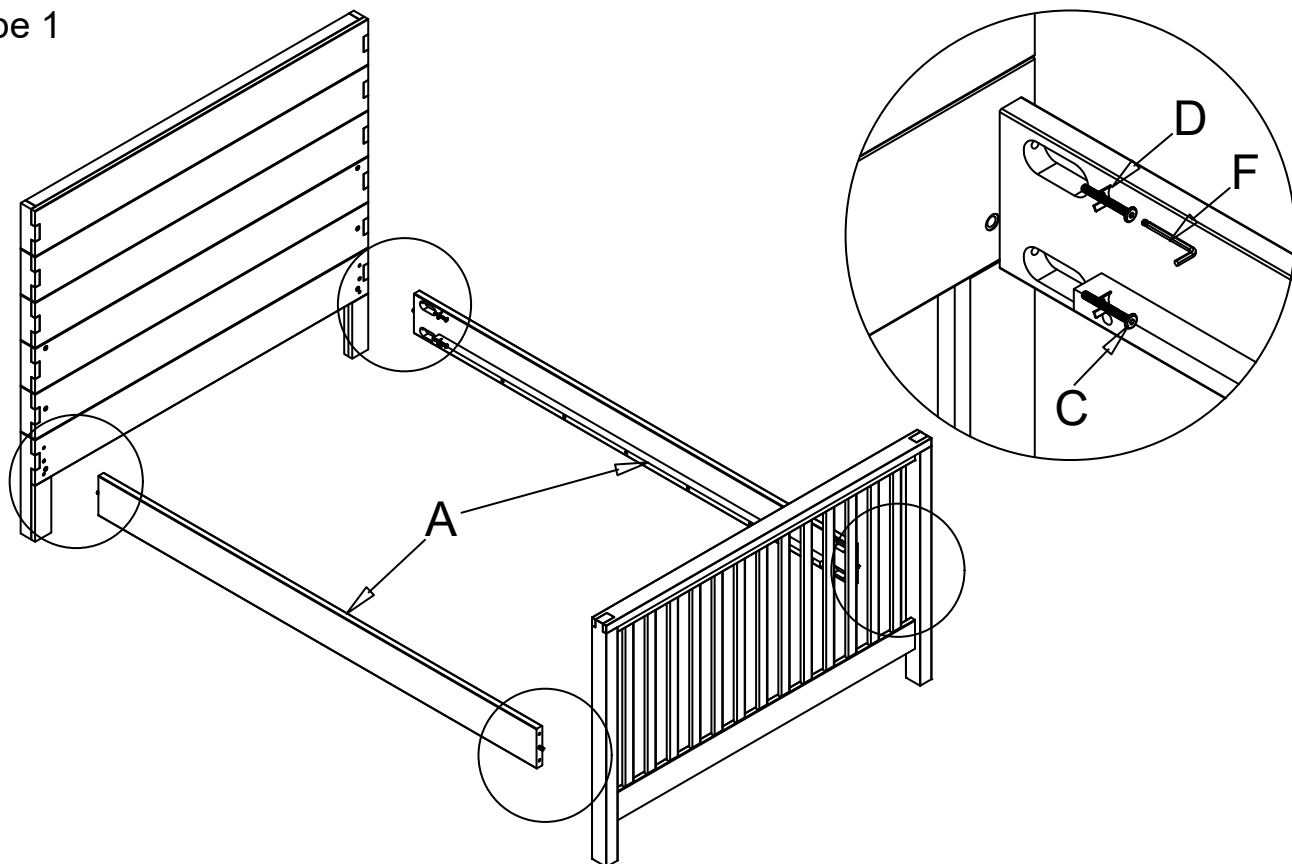
( C ) Allen Bolt 2 1/4" Boulon Allen 2 1/4" (x8)
